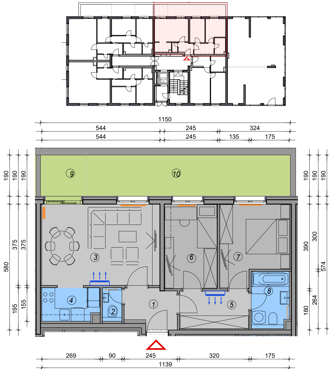
PRIZEMLJE - STAN 001 3s
